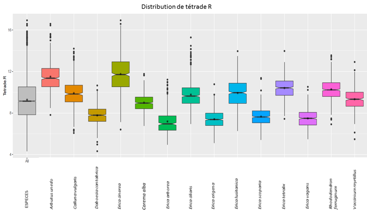
Figure 20: Distribution du rayon de la tétrade (T.R).
