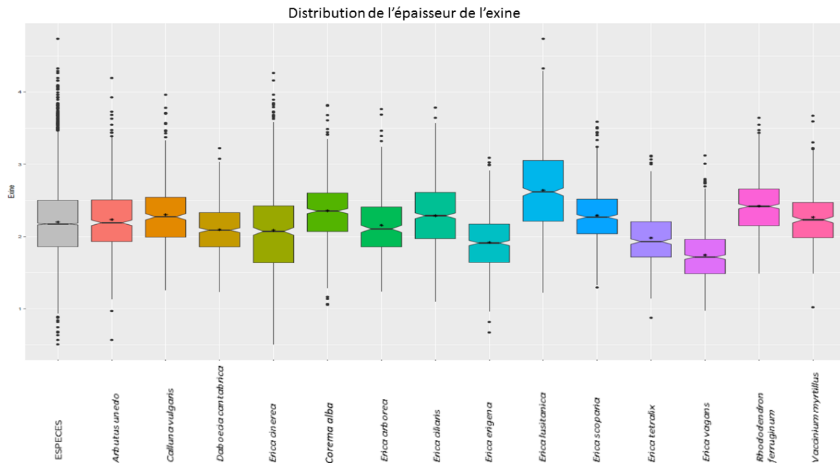
Figure 22: Distribution de l'épaisseur de l'exine (en \mu\text{m} ).
