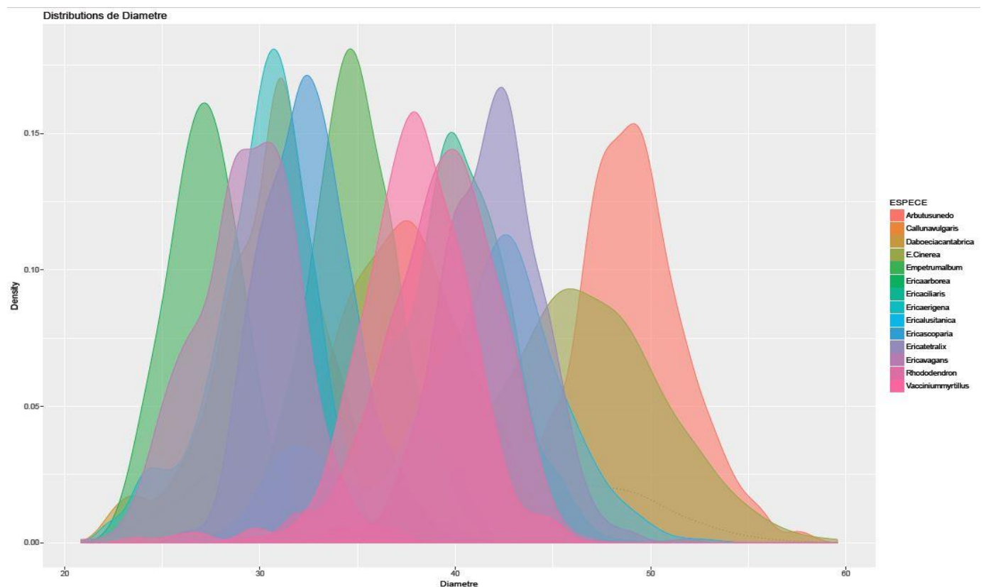
Fig 33: Courbes de distribution des diamètres des espèces
