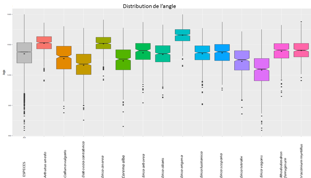
Figure 21: Distribution de l'angle entre deux tétrades.
