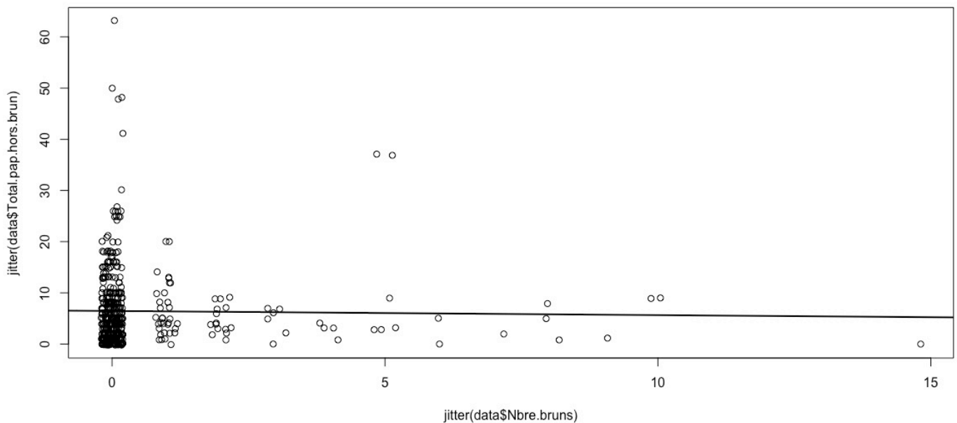
Figure 45. En haut, diversité de Rhopalocères observée en excluant le brun des pélarioniums, en fonction de l'abondance de brun des pélarioniums observé par relevé et droite de régression associée. En bas, effectifs de Rhopalocères observés en excluant le brun des pélarioniums, en fonction de l'abondance de brun des pélarioniums et droite de régression associée. La fonction jitter de R a été employée pour séparer graphiquement les points aux valeurs similaires.
