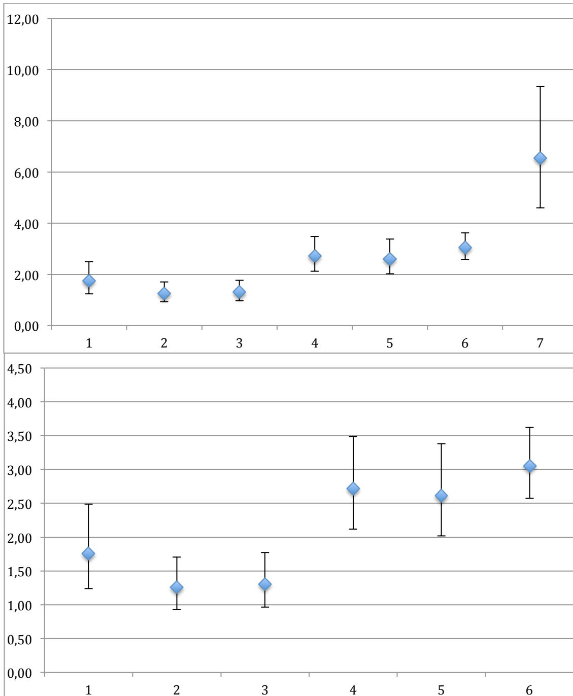
Figure 44. Données simulées par le modèle Glmer pour la diversité en Rhopalocères, excluant le brun des pélarгонiums, par classe de gestion (1 à 7 en haut, 1 à 6 en bas). Estim = estimation des moyennes par type de site avec son intervalle de confiance à 95%..
