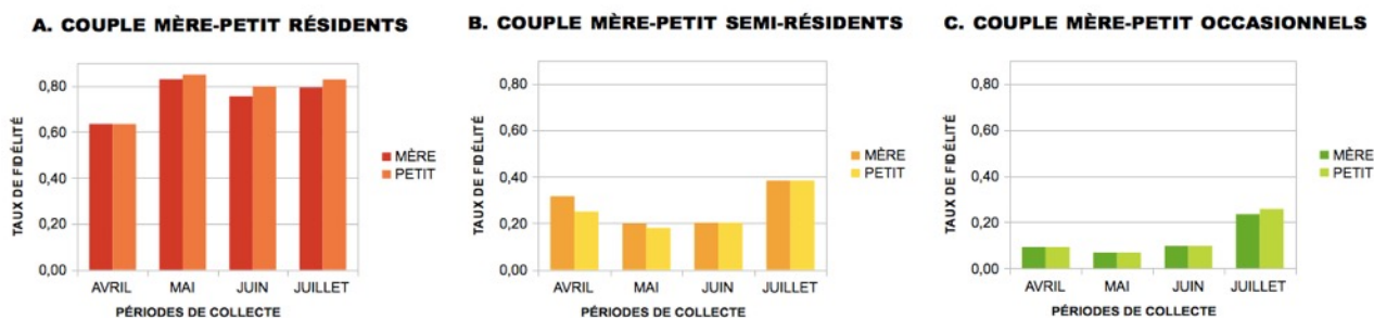
Fig. III.16. PROFILS DE TROIS COUPLES MÈRE-PETIT EN FONCTION DE LEUR DEGRÉ DE RÉSIDENCE. Profils d'un couple « résident » (A), « semi-résident » (B) et « occasionnel » (C). L'axe des abscisses représente les périodes de collecte mensuelles pour les deux saisons cumulées et l'axe des ordonnées le taux de fidélité moyen des individus sur les deux saisons.
